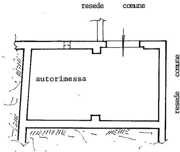
PIANO S1 - h.3,05
